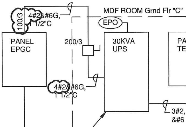
1 PARTIAL - ONE LINE RISER DIAGRAM SKE-31 SCALE: N.T.S.
