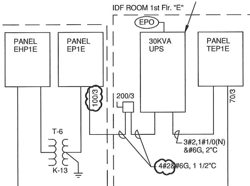
2 PARTIAL - ONE LINE RISER DIAGRAM SKE-31 SCALE: N.T.S.
